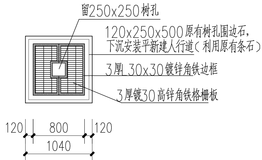
树孔平面图 1:50
