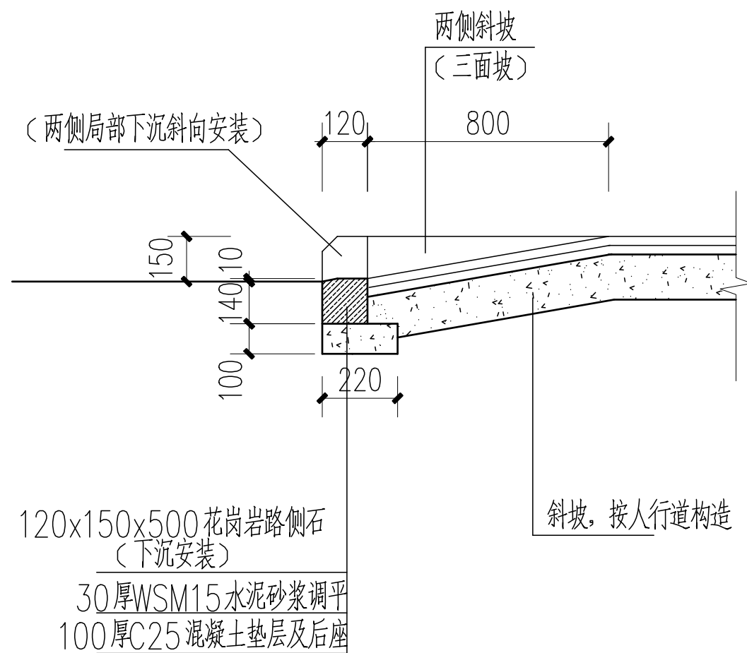
斜坡截面图 1:25
