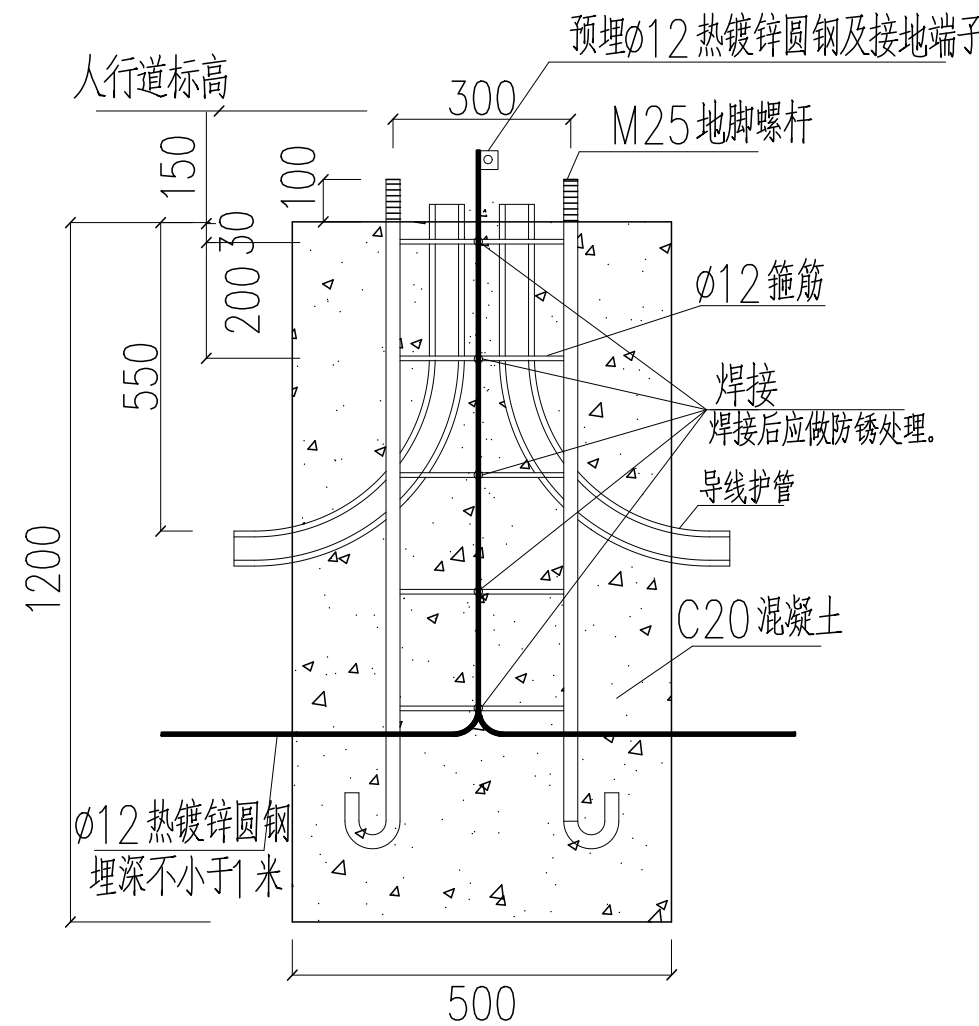
路灯基础图 1:25
