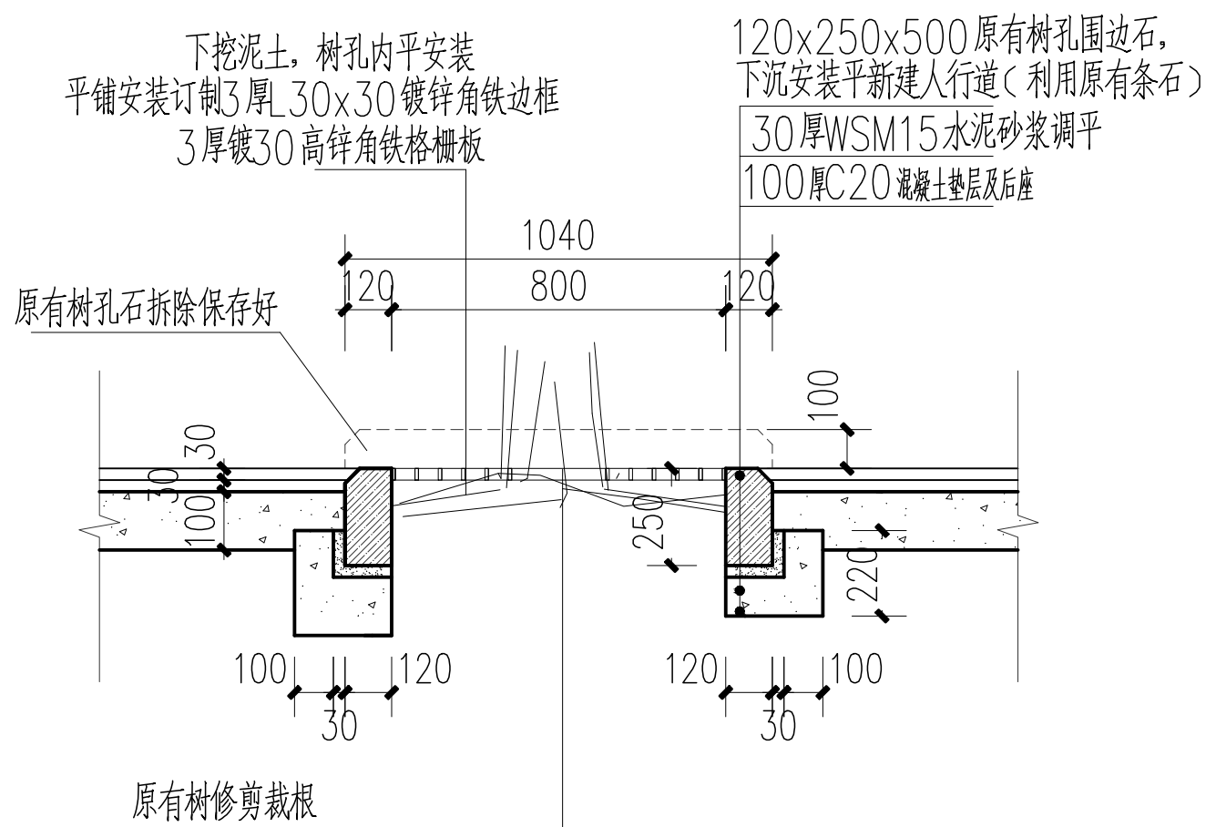
树孔截面大样图 1:25
