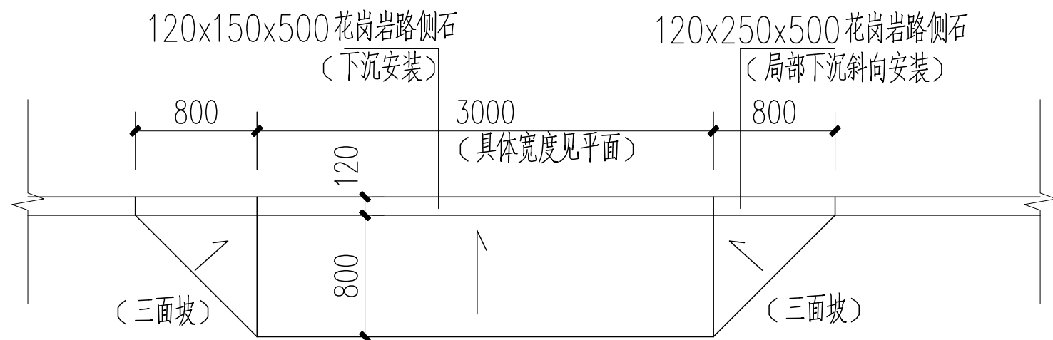
斜坡平面图 1:50
